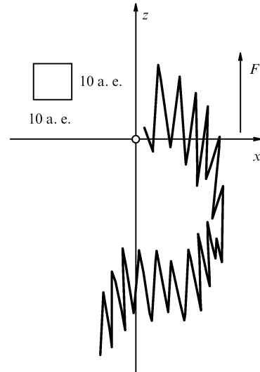
Рис. 13. Пример квазистабильной траектории для возбужденного состояния атома водорода с главным квантовым числом n = 3 , возмущаемым полем с частотой \omega = 0,15 а.е. и амплитудой напряженности F = 0,4 а.е. (линейная поляризация вдоль оси Z ). Расчет [63]
