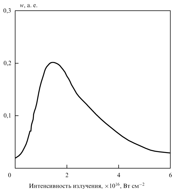
Рис. 9. Зависимость вероятности ионизации основного состояния атома водорода в единицу времени от интенсивности излучения линейной поляризации с частотой \omega = 0,65 а.е. [22]
