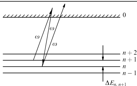
Рис. 3. Схема рамановских переходов между ридберговскими состояниями атома, отвечающая третьему порядку теории возмущений
