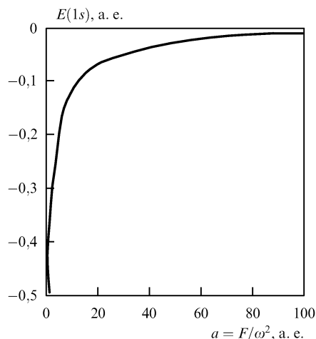
Рис. 10. Зависимость энергии основного состояния атома водорода от амплитуды колебательного движения электрона в поле линейной поляризации [32]
