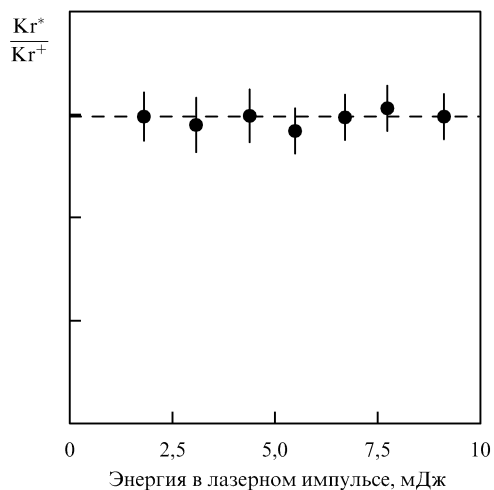
Рис. 18. Отношение числа возбужденных атомов криптона Kr^* к числу ионов криптона Kr^+ в зависимости от энергии в импульсе лазерного излучения согласно экспериментальным данным [83]
