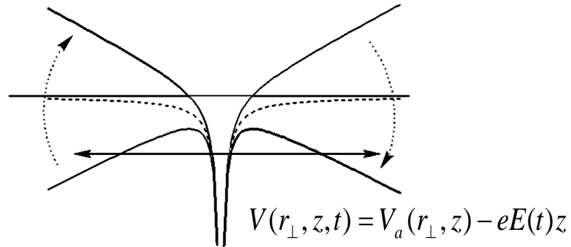
Атомный потенциал при наличии сильного лазерного поля
