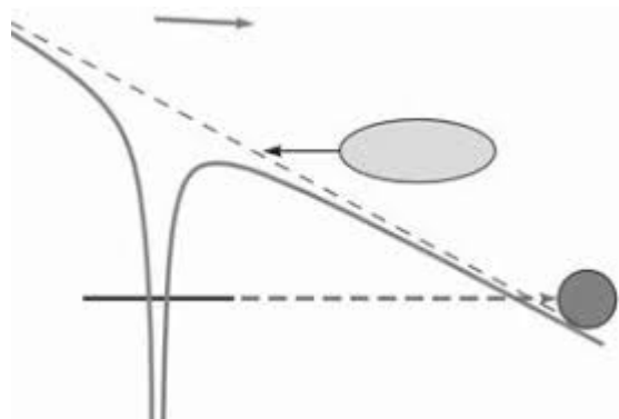
Эффект перерасеяния (P. Corkum, 1993)
